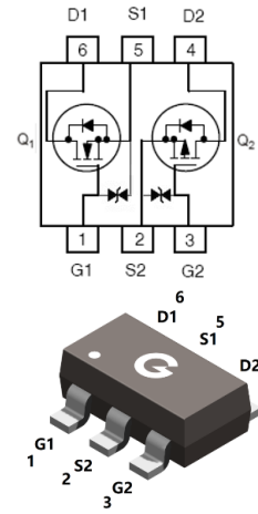
SOT-23-6L
