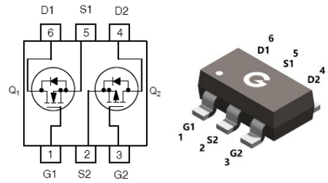
SOT-23-6L
